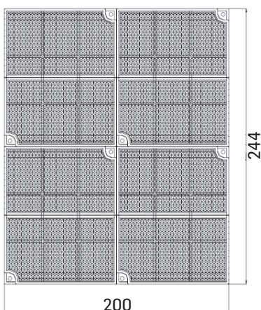
Fig.10b(unit: mm)
